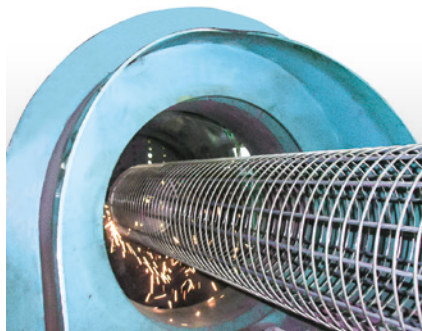
点溶接状況
