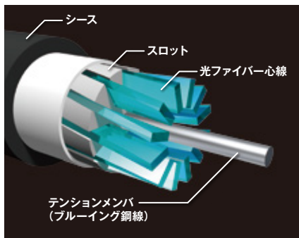
スロット型光ケーブル断面図
